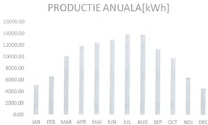
Fig. 6 - Curba de producție anuală
