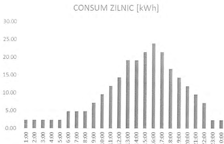
Fig. 1 - Curba de consum zilnica
