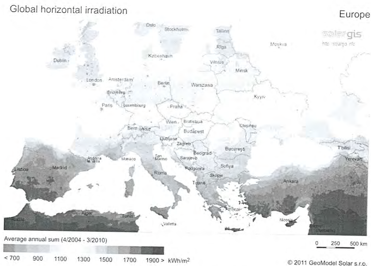
Fig. 8 – Harta radiației solare în Europa
